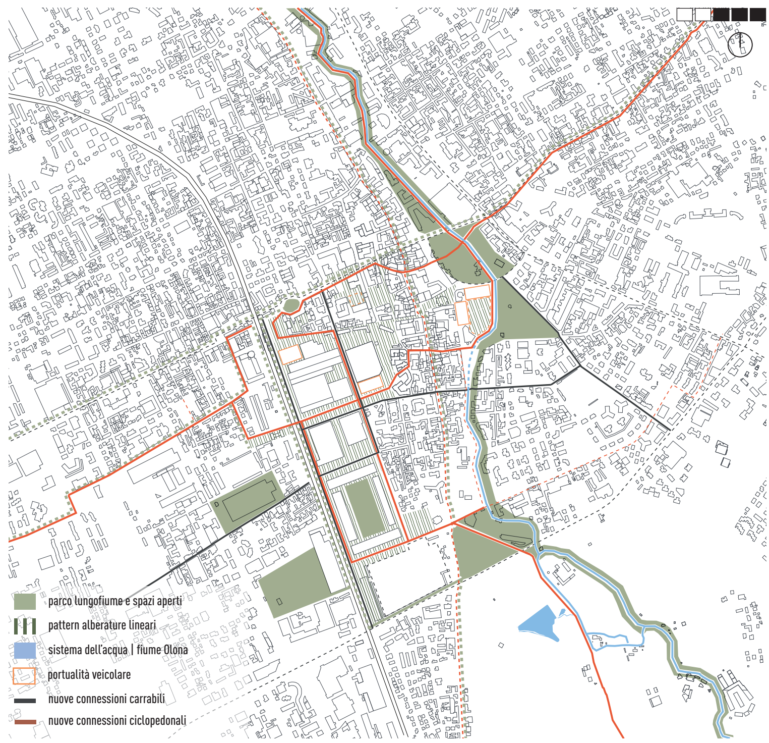
SdP Stato di Progetto | MASTERPLAN Rete Tessuto
