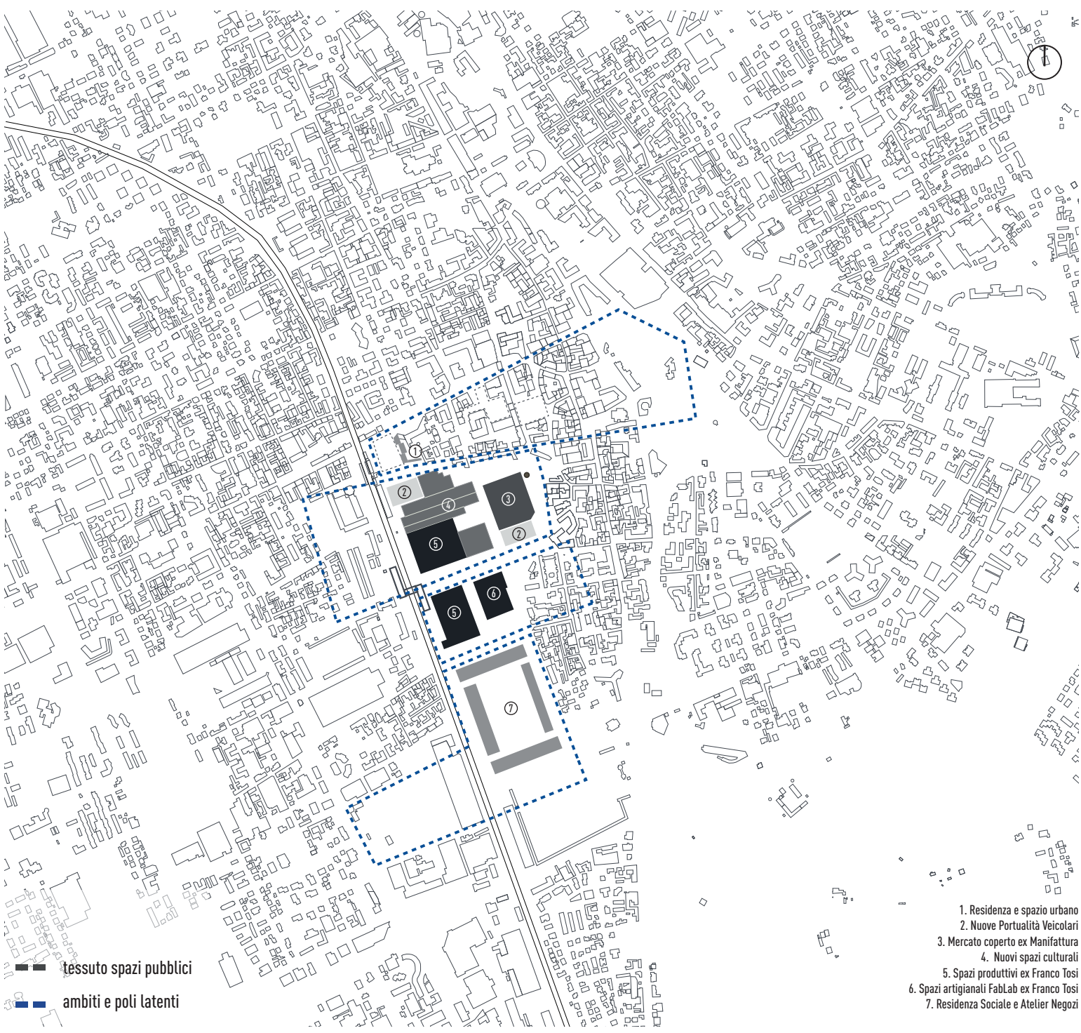
SdP Stato di Progetto | MASTERPLAN Connessione Riuso
